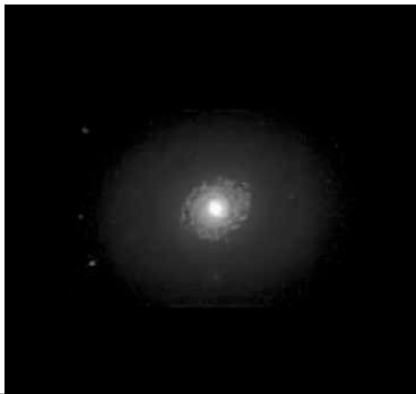
Visible - 1 (KPNO)
