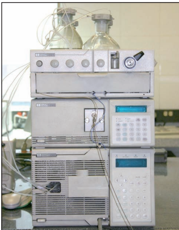
Cromatógrafo líquido de alta eficiencia.
