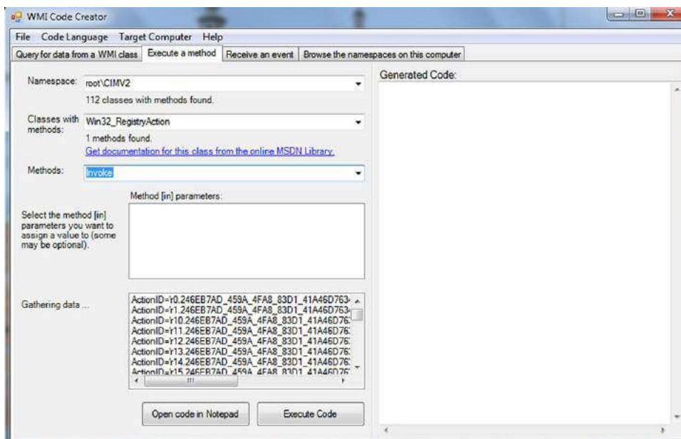
Fig. 2.7. WMI (III)
