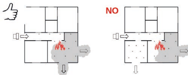
Imagen 140. Dos aperturas en el recinto de incendio contribuyen a la evacuación de gases de forma conjunta mientras que dos aperturas en distintos recintos debilitarán el flujo principal necesario en el recinto de incendio
