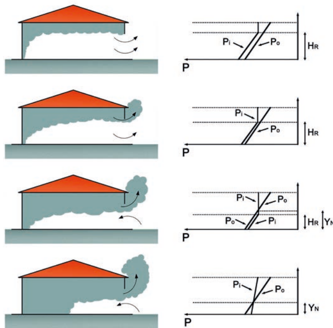
Imagen 64. Variación de la presión dentro de un incendio interior con apertura al exterior a lo largo de las distintas fases de desarrollo
