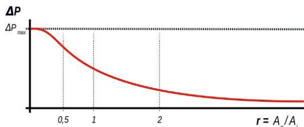
Imagen 143. Variación del diferencial de presión interior ( \Delta P ) y la relación ( r ) entre la salida de gases ( A_e ) y la entrada ( A_i )
