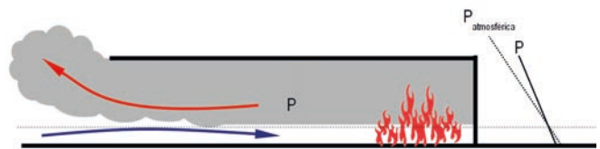
Imagen 57. Flujo bidireccional junto a una representación de la variación de los valores absolutos de presión atmosférica (línea de puntos) y presión interior (línea continua) con respecto a la altura
