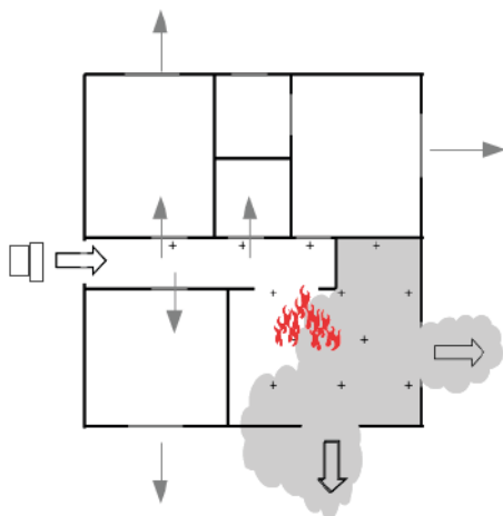
Imagen 144. El mal sellado de la estructura genera pérdidas de flujo e ineficiencia. Esto dificulta especialmente las operaciones con técnicas de Ventilación VPP Ofensiva
