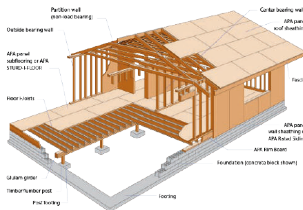
Imagen 163: Estructura de entramado ligero
