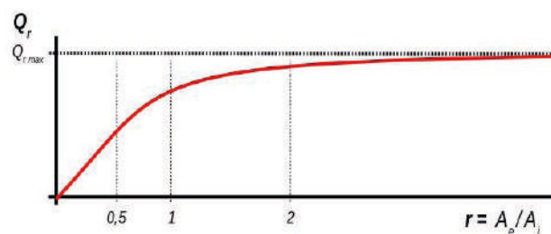
Imagen 142. Variación del caudal efectivo ( Q_r ) y la relación ( r ) entre la salida de gases ( A_e ) y la entrada ( A_i ). Una salida dos veces el tamaño de la salida da resultados más que suficientes
