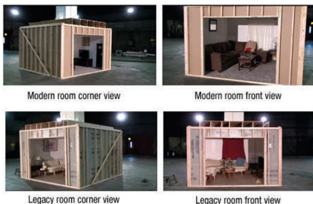
Imagen 5. Detalle de la configuración del experimento de comparación de combustible moderno y tradicional
