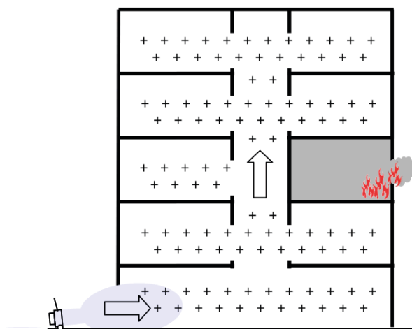
Imagen 71. Presurización de un bloque de viviendas para evitar la propagación y dispersión de gases. Obsérvese que el recinto permanece lo más cerrado posible para evitar pérdidas de flujo y por tanto de presión interior
