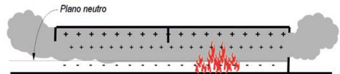
Imagen 13. Esquema de posición del plano neutro. Los signos (+) y (-) indican diferenciales de presión positivos y negativos respectivamente sobre la presión exterior
