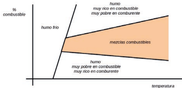
Imagen 38. Gráfica de variación del rango de inflamabilidad de un combustible con relación a la temperatura
