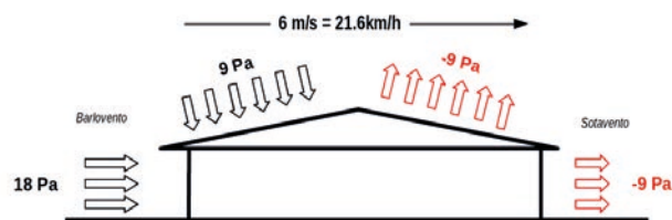
Imagen 149. El diferencial de presión generado en cada una de las fachadas.
