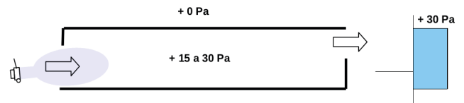
Imagen 68. Distribución de diferenciales de presión en un recinto sometido a ventilación VPP
