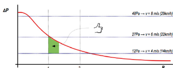
Imagen 152. Saldo de presión interior en una técnica de VPP en contra del viento
