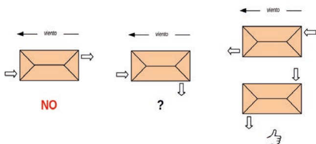
Imagen 150. Las configuraciones en las que entrada o salida reciben una presión eólica contraria al flujo que se quiere establecer deben ser evitadas
