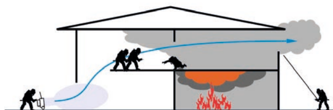
Imagen 120. La Ventilación en Presión Positiva Defensiva se basa en el confinamiento del incendio para evacuar los gases de incendio del resto de la estructura
