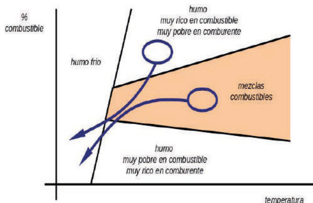
Imagen 43. Efecto de enfriamiento y dilución mediante aplicación de agua
