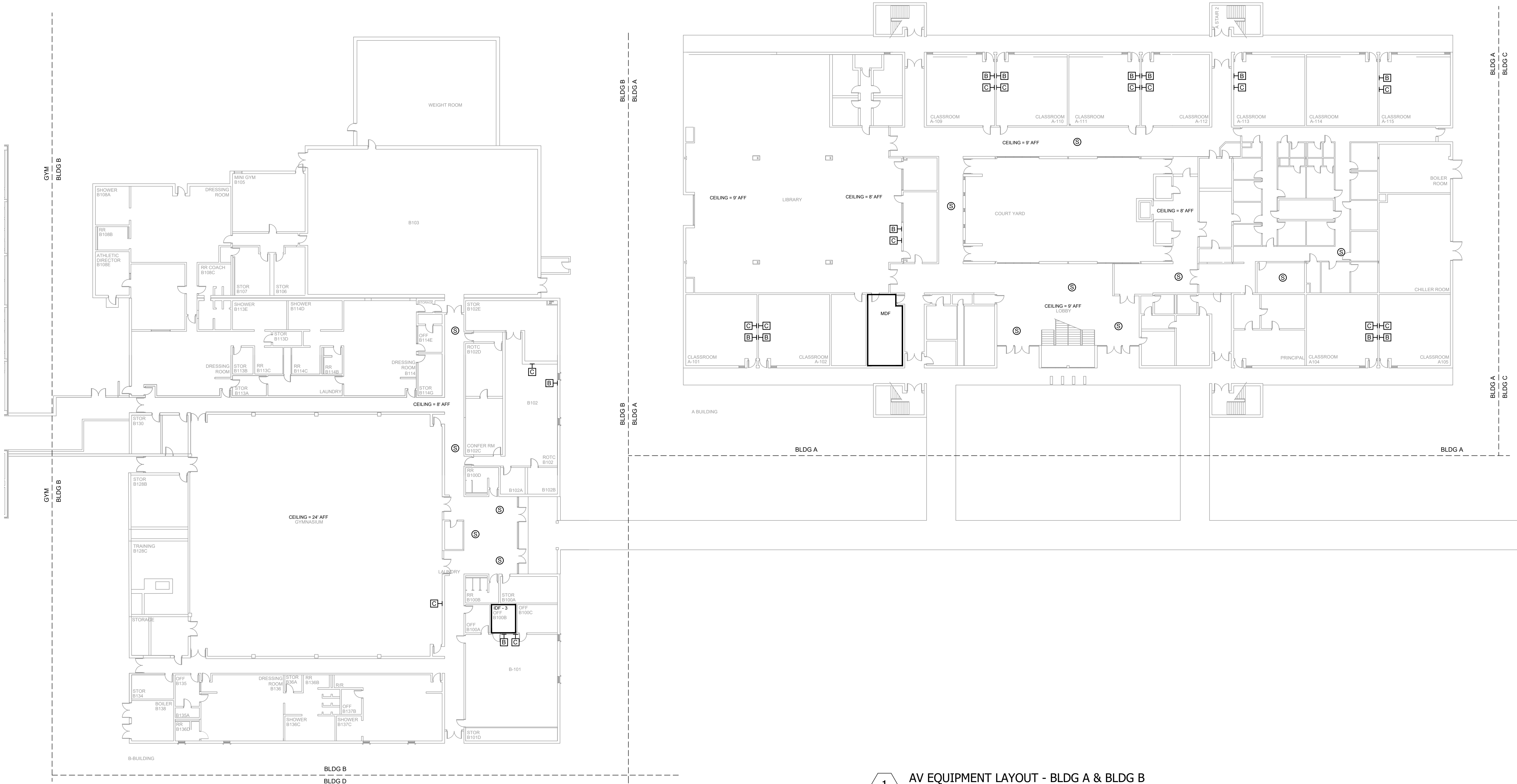
1 AV EQUIPMENT LAYOUT - BLDG A & BLDG B SCALE: NTS
