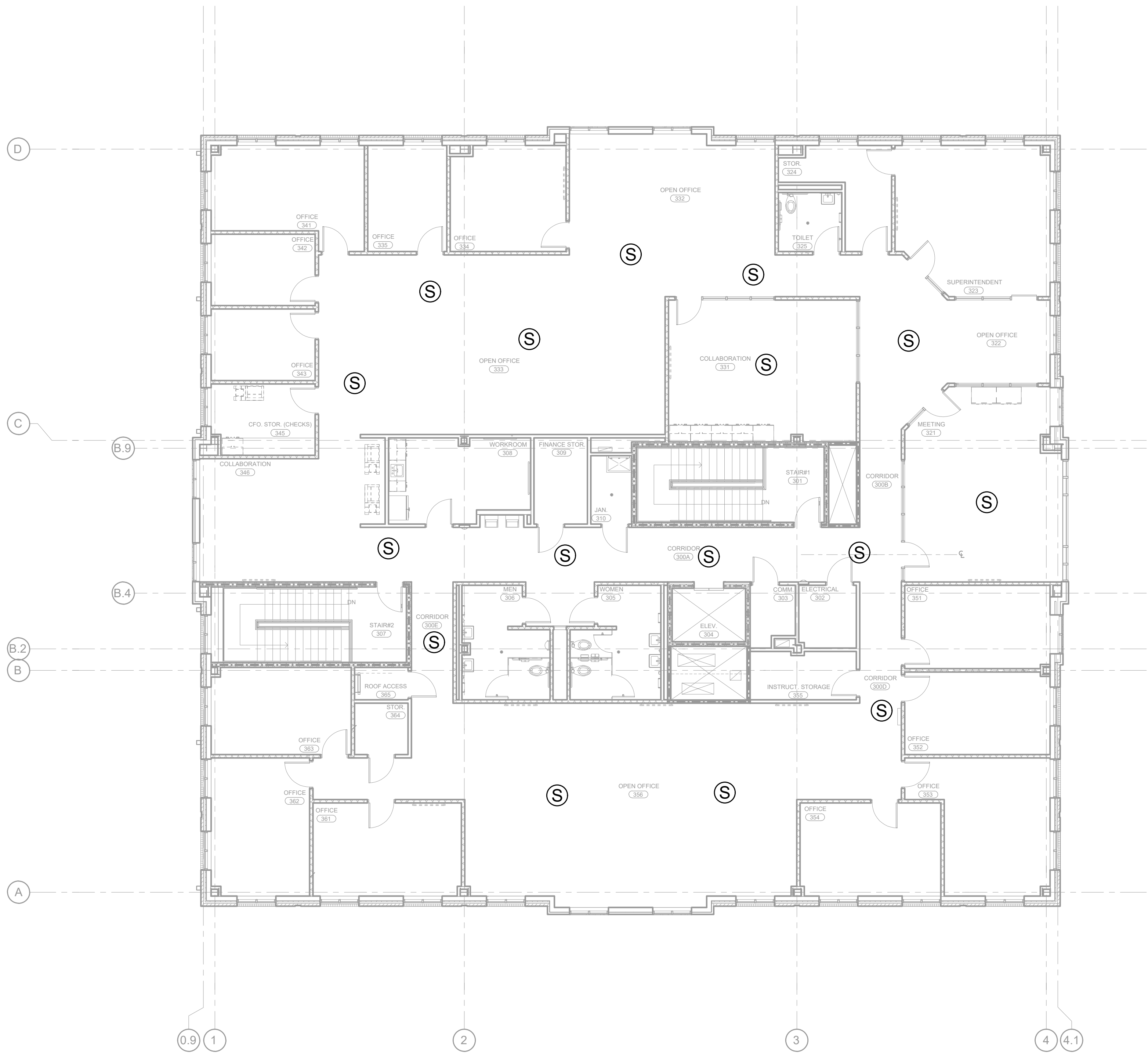
1 AV EQUIPMENT LAYOUT SCALE: NTS
