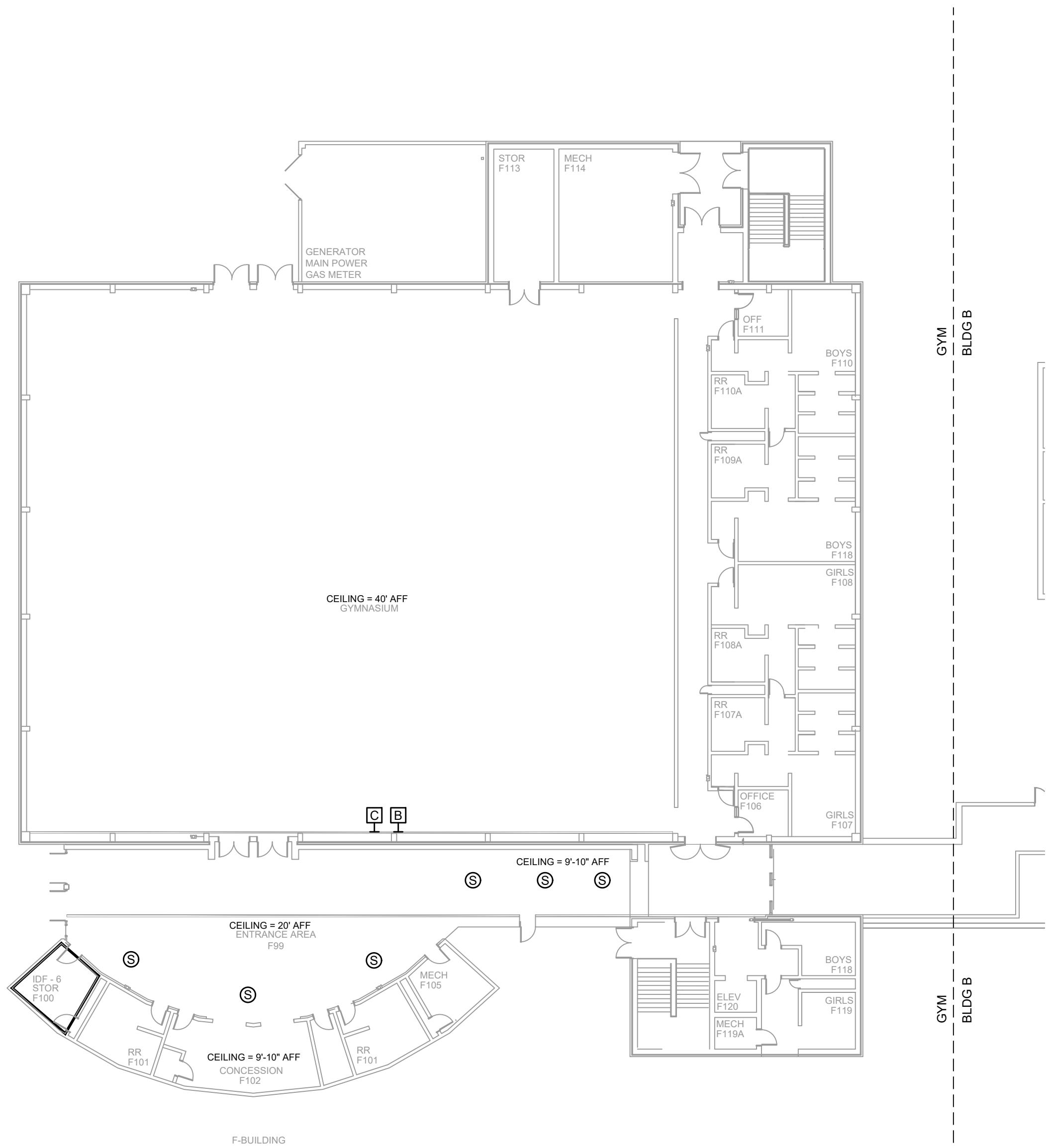
1 AV EQUIPMENT LAYOUT - GYM SCALE: NTS
