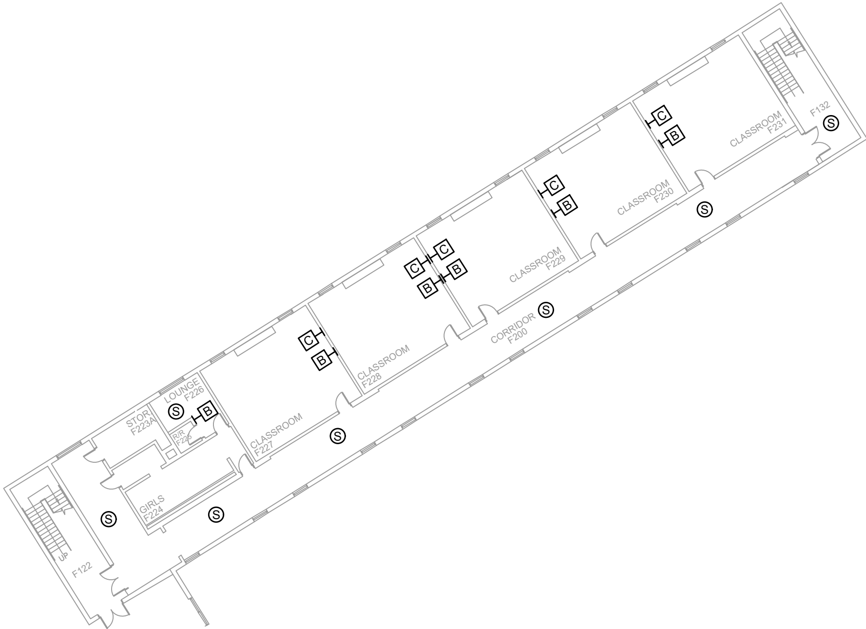
1 AV INFRASTRUCTURE LAYOUT - 2ND FLOOR SCALE: NTS
