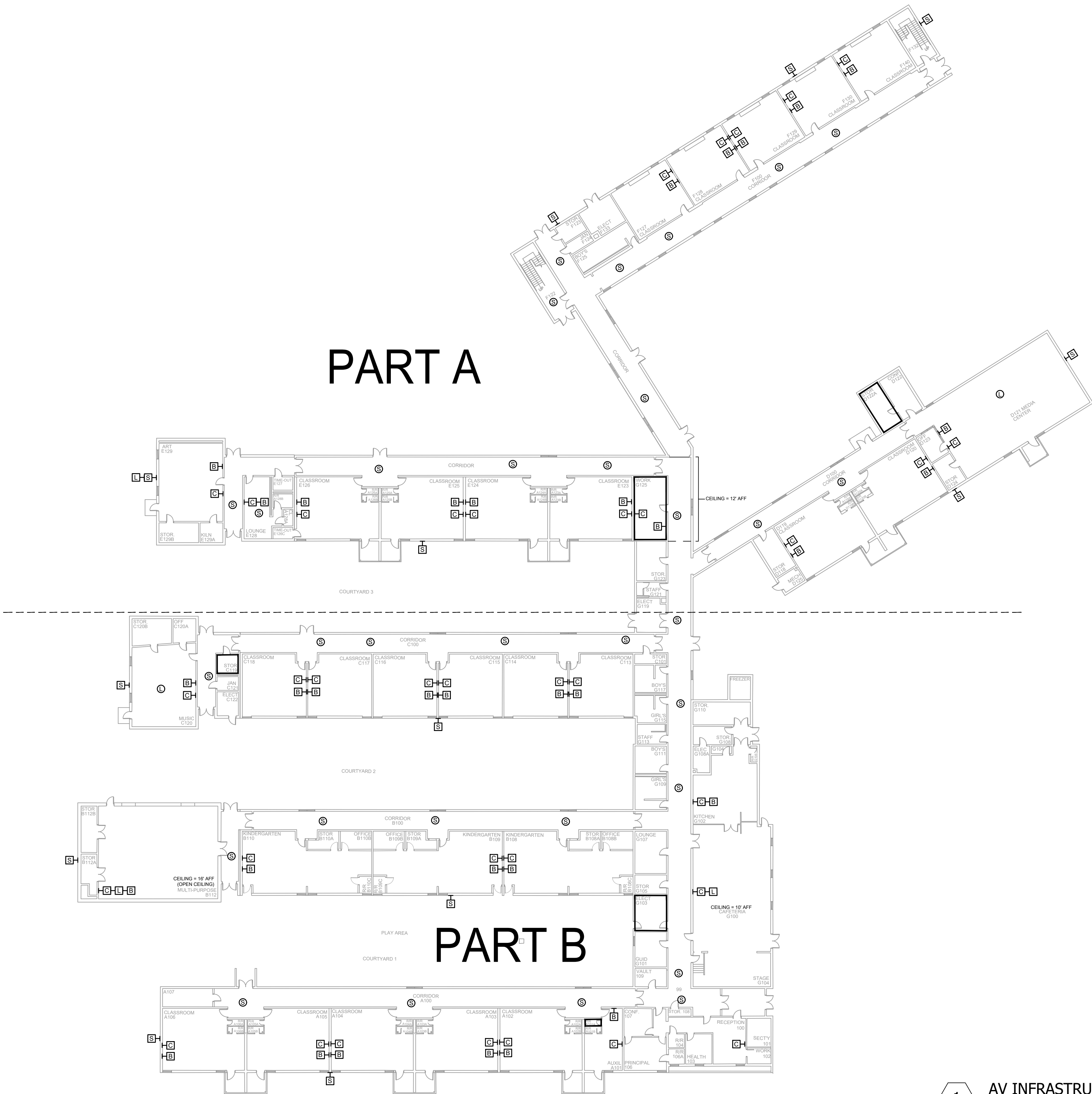
1 AV INFRASTRUCTURE LAYOUT - OVERALL SCALE: NTS
