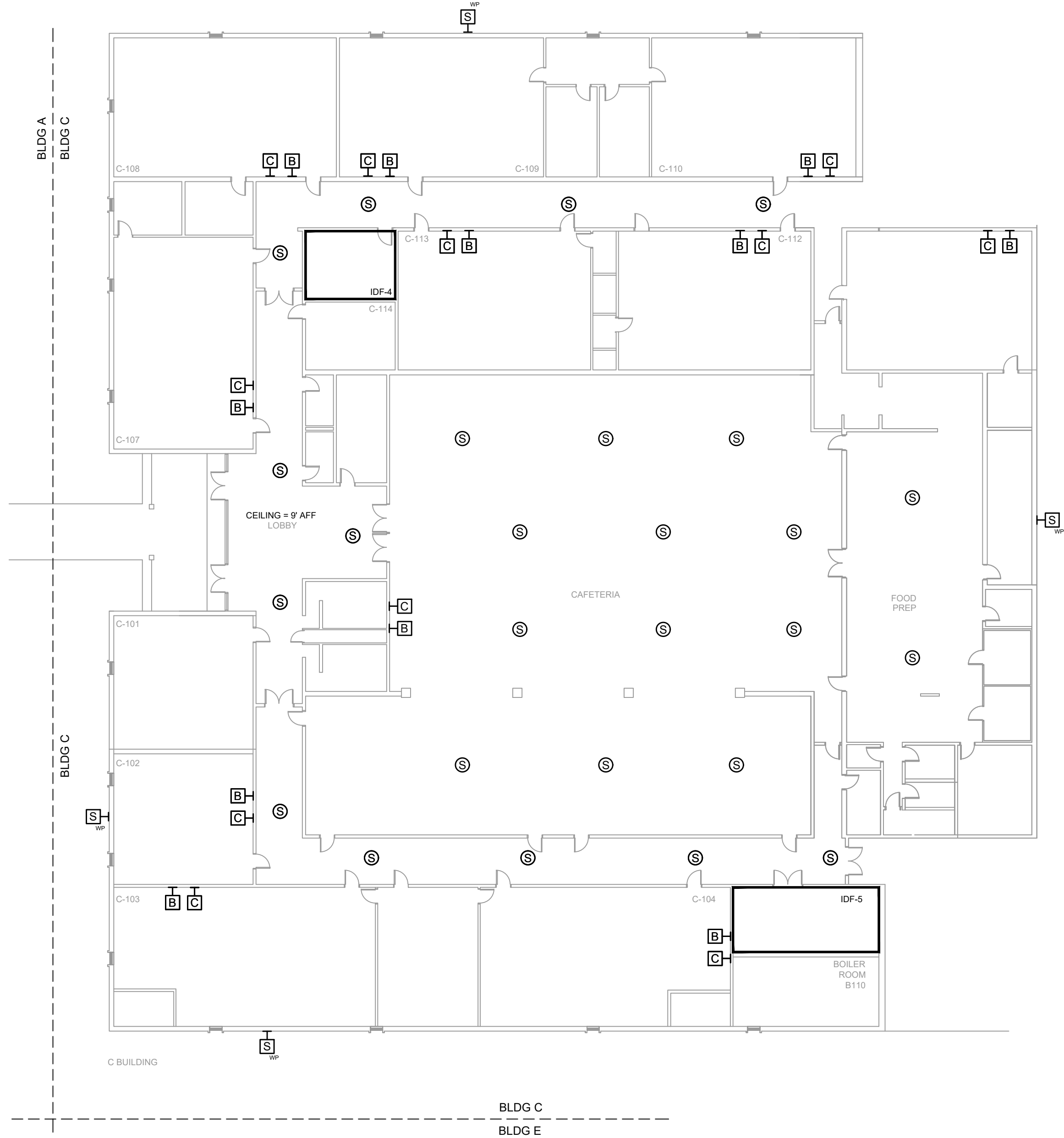
2 AV EQUIPMENT LAYOUT - BLDG C SCALE: NTS
