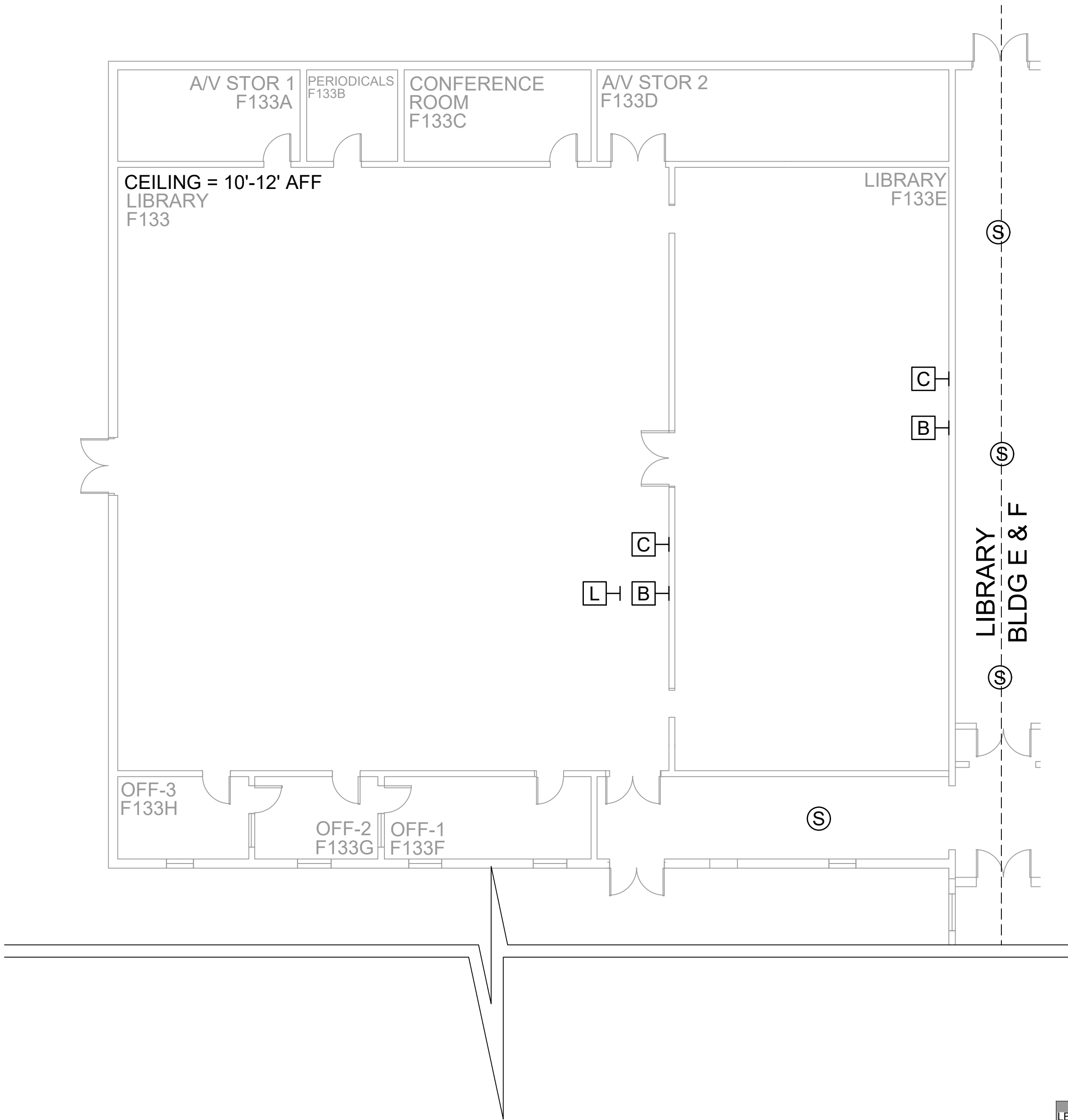
2 AV EQUIPMENT LAYOUT - LIBRARY SCALE: NTS
