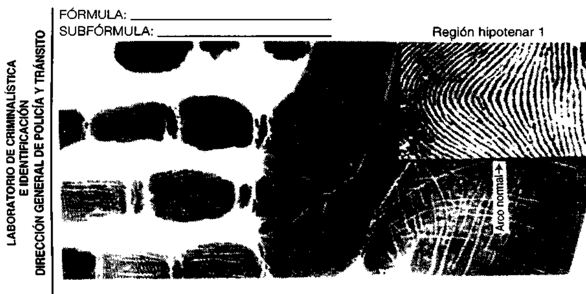
Figura 3.28. Arco normal
