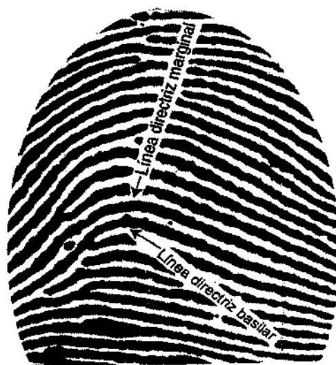
Figura 1.42. Arco normal
