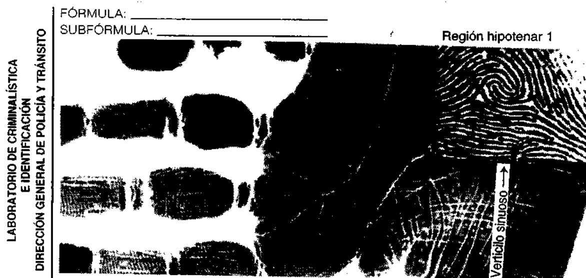
Figura 3.34. Verticilo sinuoso
