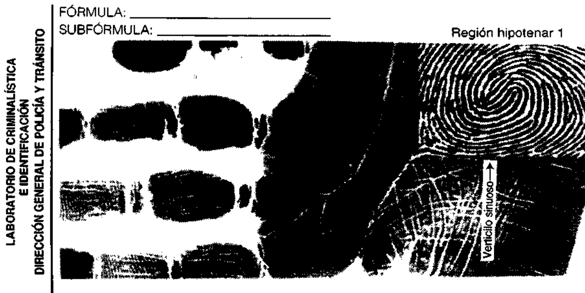
Figura 3.25. Verticilo sinuoso
