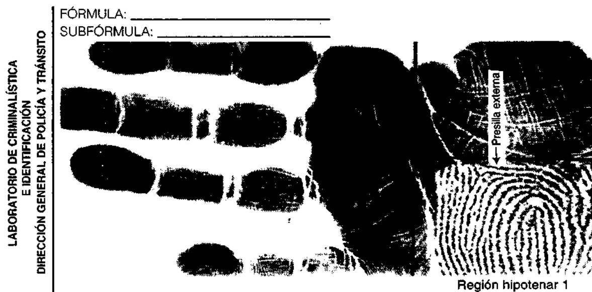
Figura 3.24. Presilla externa
