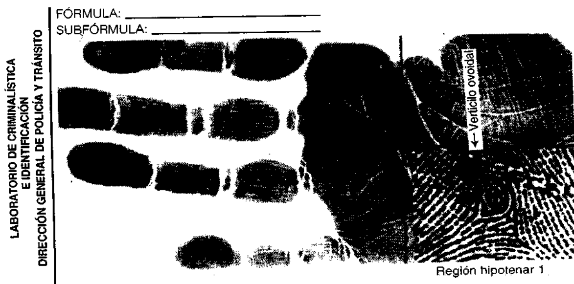
Figura 3.35. Verticilo ovoidal
