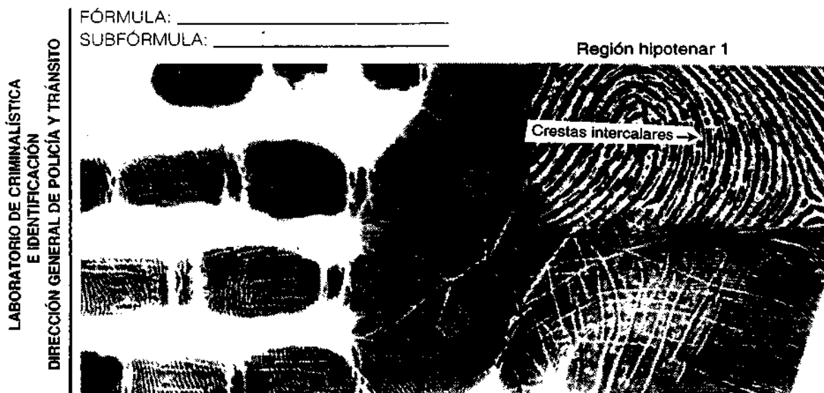
Figura 3.12. Crestas intercalares
