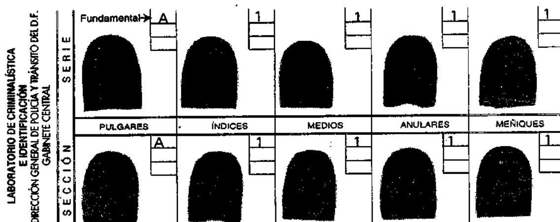
Figura 1.60. Fórmula dactiloscópica
