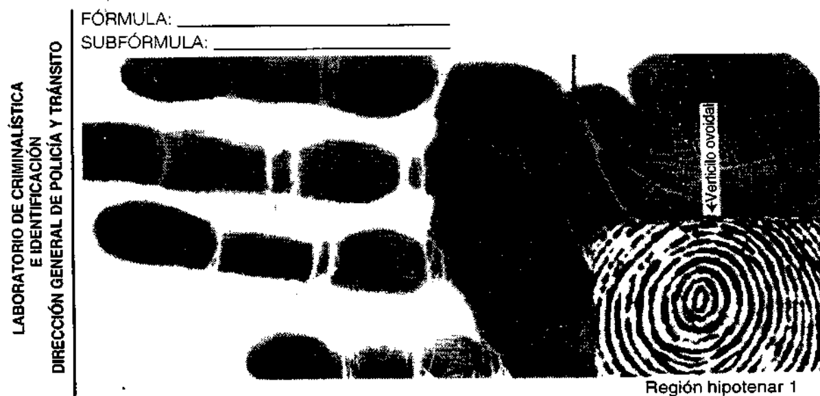
Figura 3.47. Verticilo ovoidal
