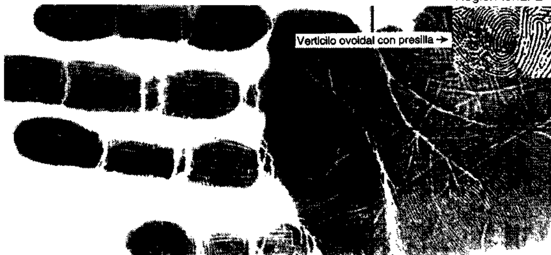
Región tenar 2
