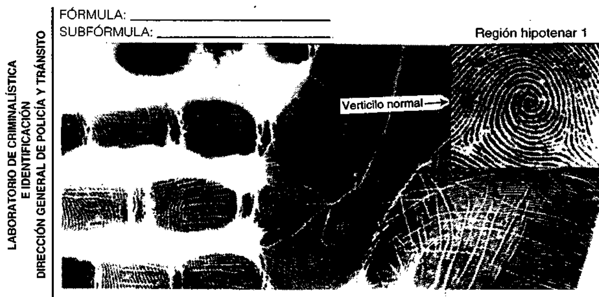
Figura 3.27. Verticilo normal
