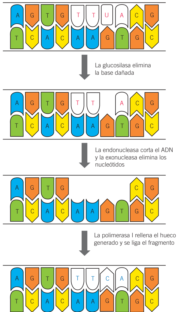
Figura 9-4. Reparación por escisión de bases.
