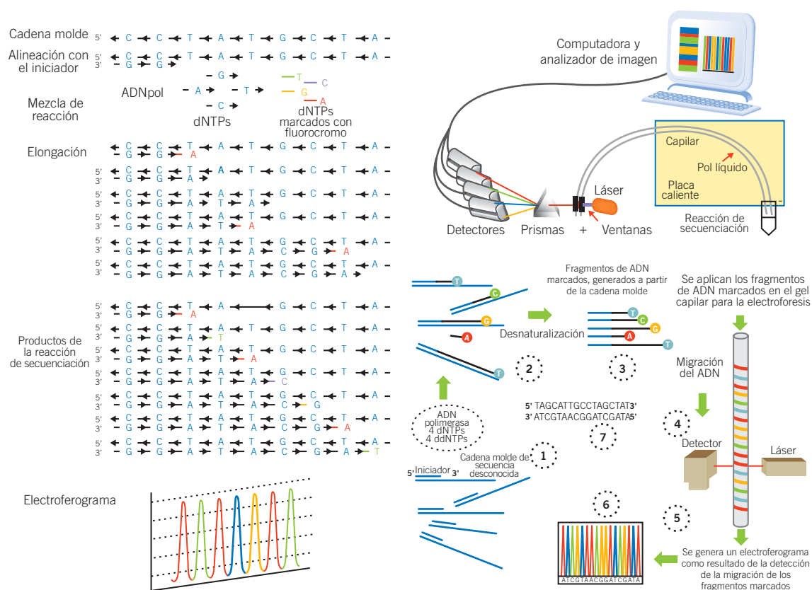
Figura 17-4. Método de secuenciación automatizado. Para realizarlo se obtienen fragmentos de ADN de la hebra molde de interés, se marcan los cuatro nucleótidos con fluorocromo de distinto color, se realiza el ciclo de secuenciación mediante PCR, se eliminan NTP sobrantes. Los fragmentos son sometidos a electroforesis en gel y mediante el sistema automatizado; el láser emitirá la luz que el detector interpreta diferencialmente de acuerdo con el fluorocromo que pase por el haz de luz para generar un patrón de curvas de acuerdo a la longitud de onda diferente para cada base, a fin de poder leer la secuencia obtenida.
