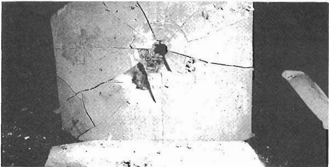
Impacto de un proyectil del calibre 7.62x 63 mm (.30-06) sobre una placa de cerámica del nivel IV
