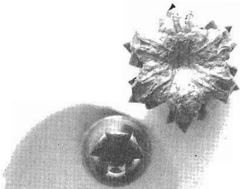
Cartucho con proyectil Black Talon
