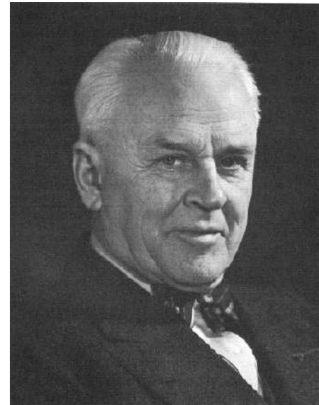
Robert Millikan
