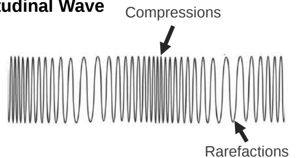
Longitudinal Wave
