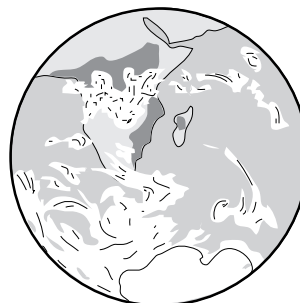
Earth 1X
