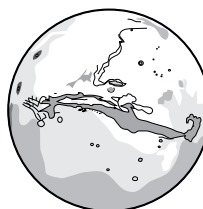
Mars 0.53X
