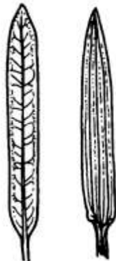
LINEAR
