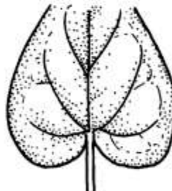
CORDATE
