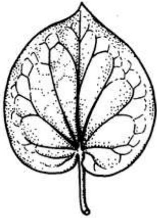
CORDATE
