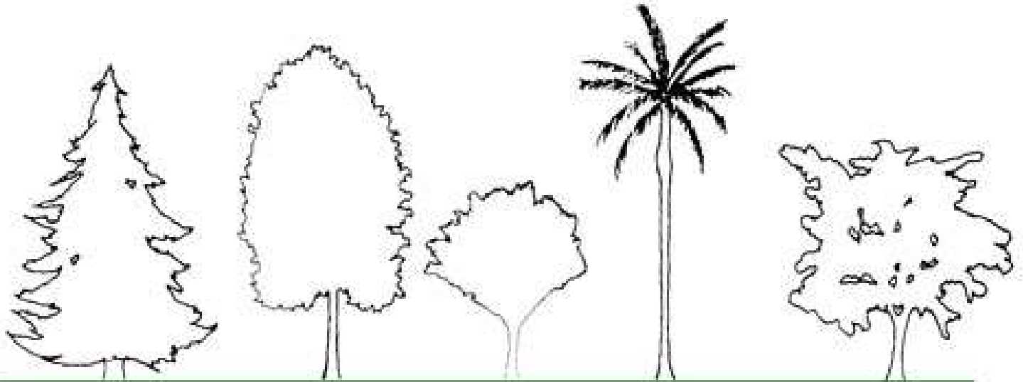
Pyramidal
