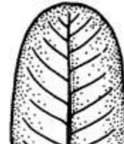
OBTUSE
