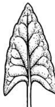
SAGITTATE
