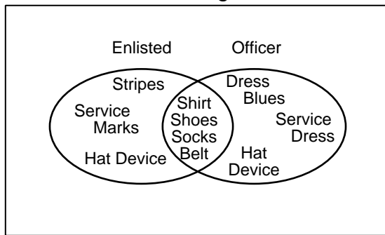
Venn Diagram
